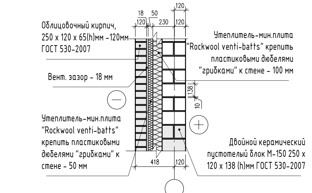
КОНСТРУКТИВНОЕ РЕШЕНИЕ НАРУЖНОЙ СТЕНЫ ИЗ ДВОЙНОГО КЕРАМИЧЕСКОГО БЛОКА С ОБЛИЦОВКОЙ КИРПИЧОМ • М 1:25
